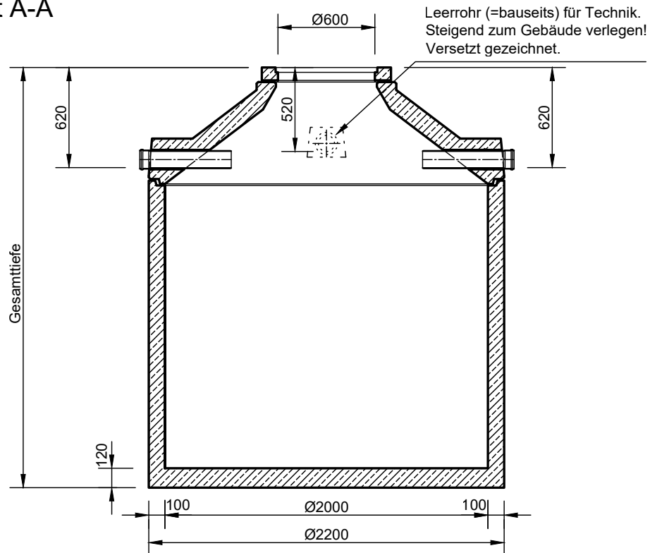
Schnitt A-A
