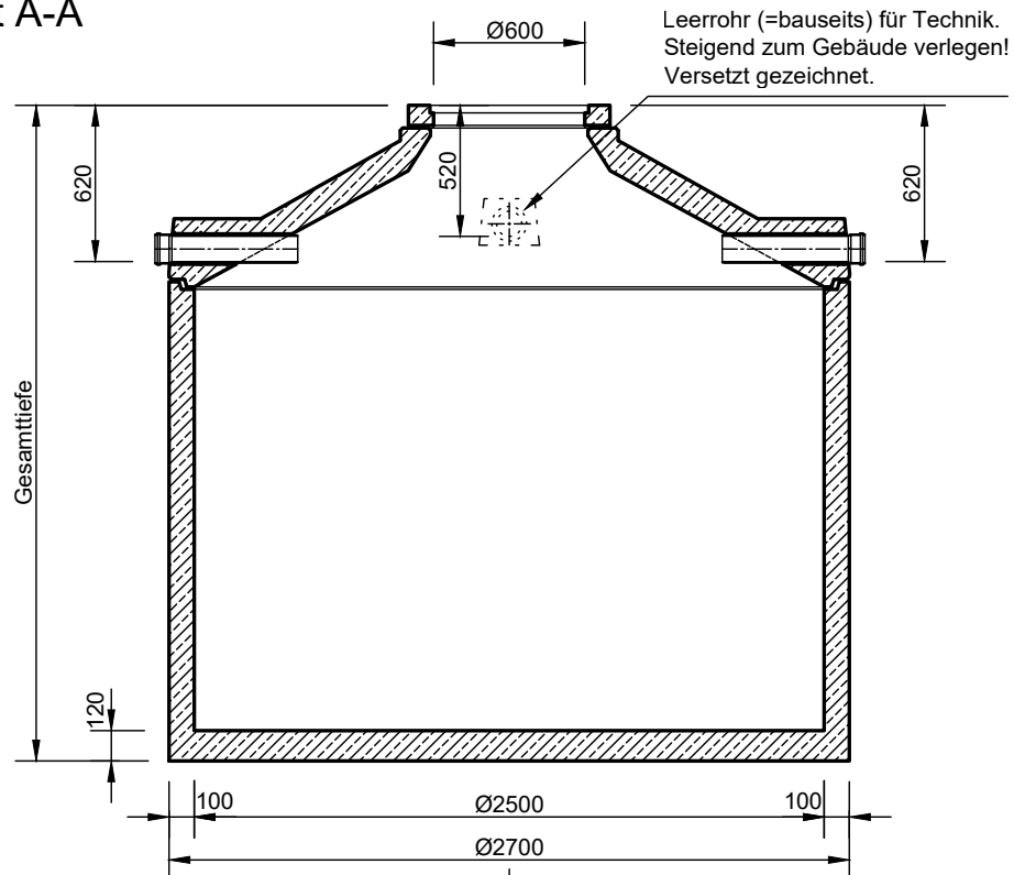
Schnitt A-A
